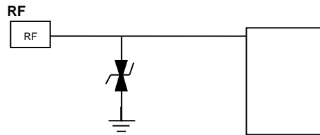
ESDULC5V0D8B
